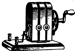
FIG. 281.—A magneto.
