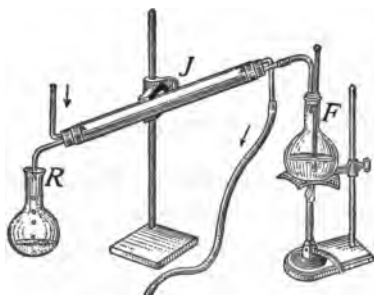
FIG. 155.—Distilling apparatus.
