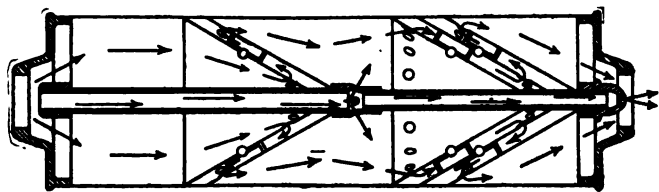
FIG. 166.—An efficient automobile muffler.
