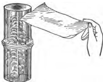
FIG. 6.—Diffusion of gases.
