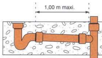
Figure 24 : Le passage des évacuations dans les parois
