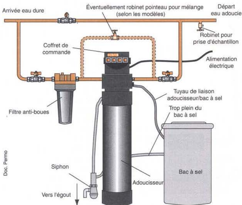
Figure 15 : L'adoucisseur
