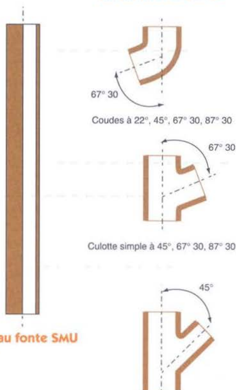
Embranchements simples à 45°, 67° 30'
