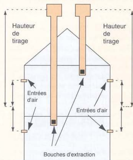
Figure 64 : La hauteur de tirage
