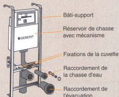
En applique avec habillage léger (bois, plaque de plâtre)
