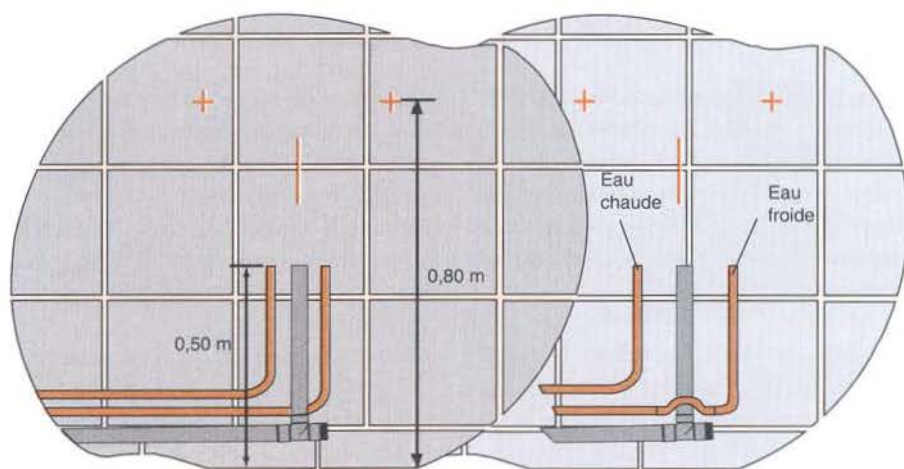
Figure 118 : La mise en attente des canalisations d'un lavabo
