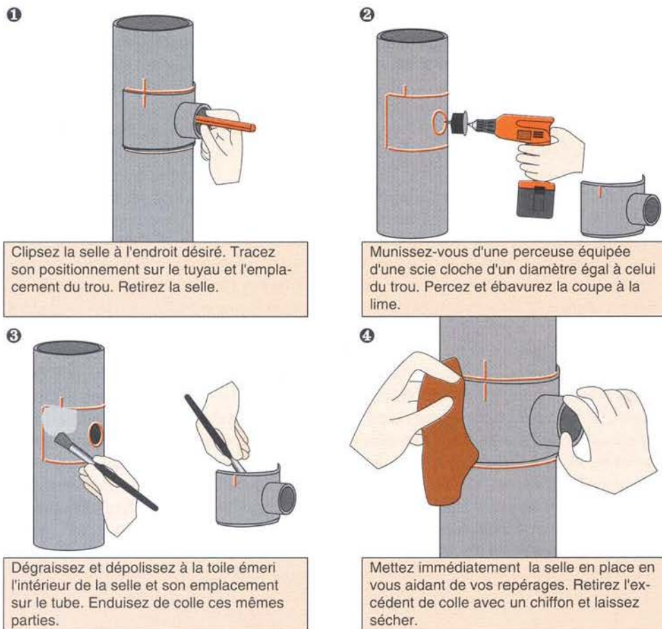
Figure 95 : La pose d'une selle de branchement
