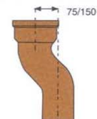
Coude d'étage
