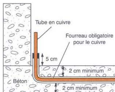
Parcours encastré en dalle béton (avant la réalisation de la dalle, puisque l'engravure est interdite dans une dalle existante)
