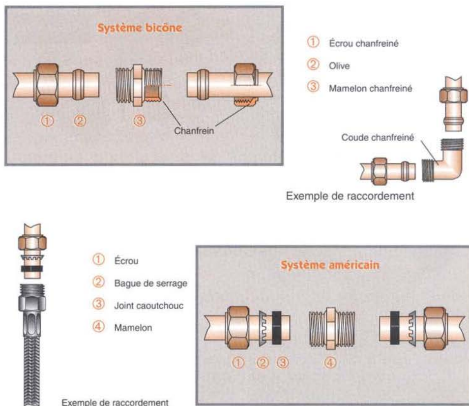
Figure 103 : Les raccords sans soudure
