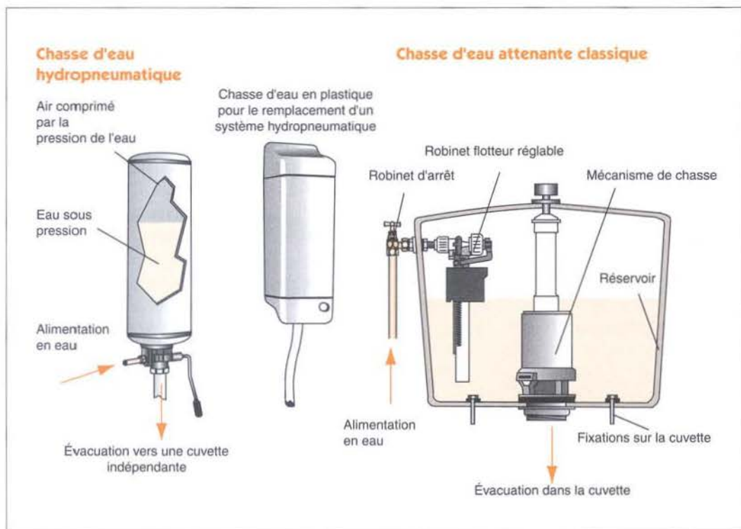
Figure 56 : Les chasses d'eau
