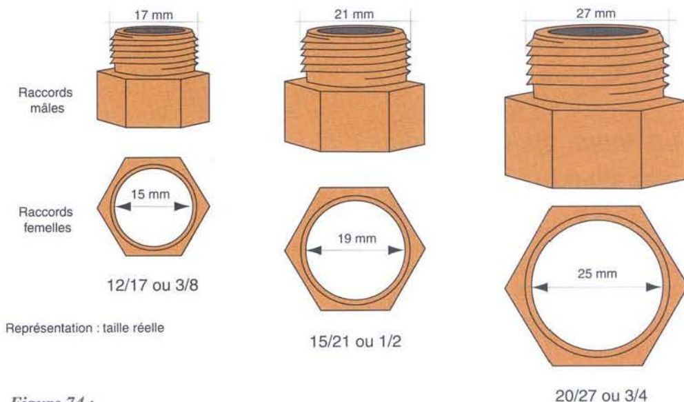
Figure 74 : Les principaux filetages utilisés
