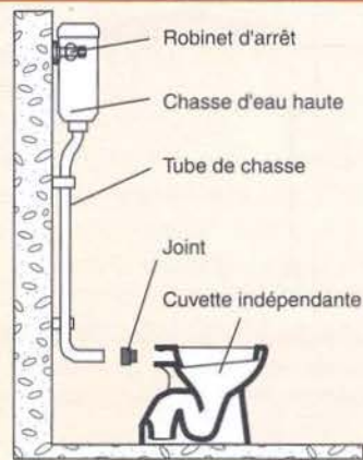
Raccordement d'une chasse d'eau haute
