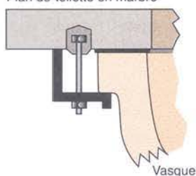
Figure 53 : Les vasques à recouvrement et à encastrer
