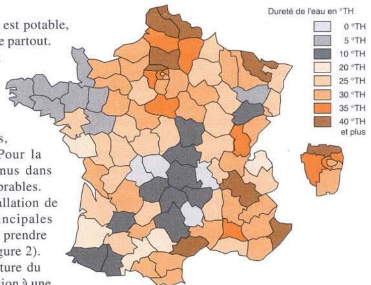
Figure 2 : La carte de la dureté de l'eau
