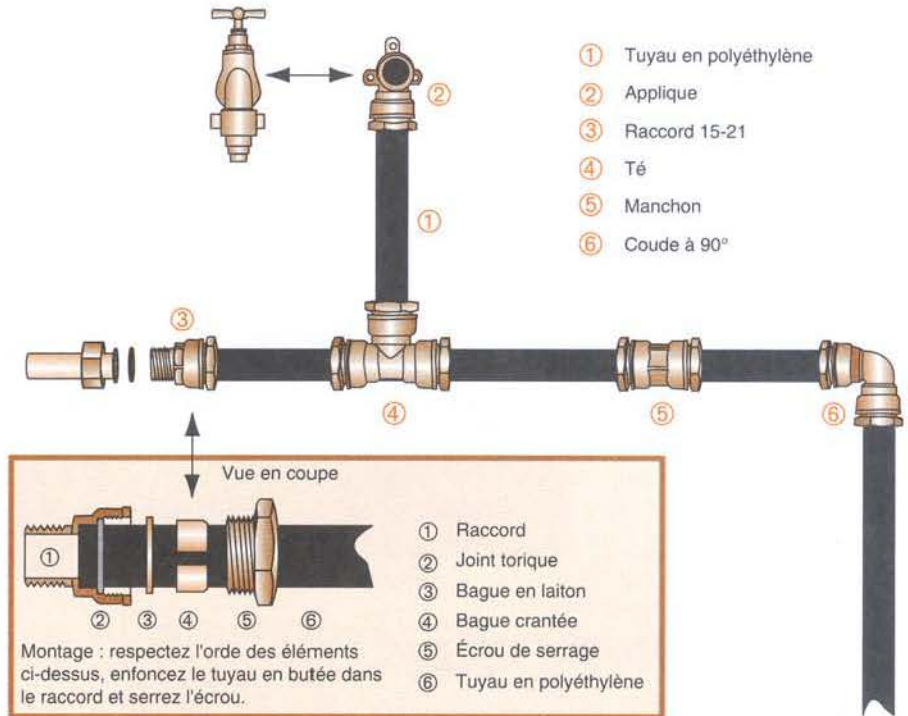
Figure 98 : Les raccords et l'assemblage des tuyaux en polyéthylène
