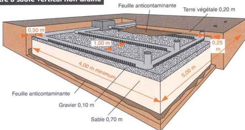
Figure Les systèmes filtre à
