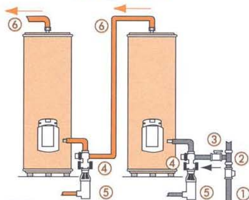
Figure 144 : Les divers raccordements hydrauliques
