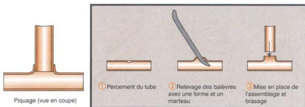
Figure 109 : Le piquage
