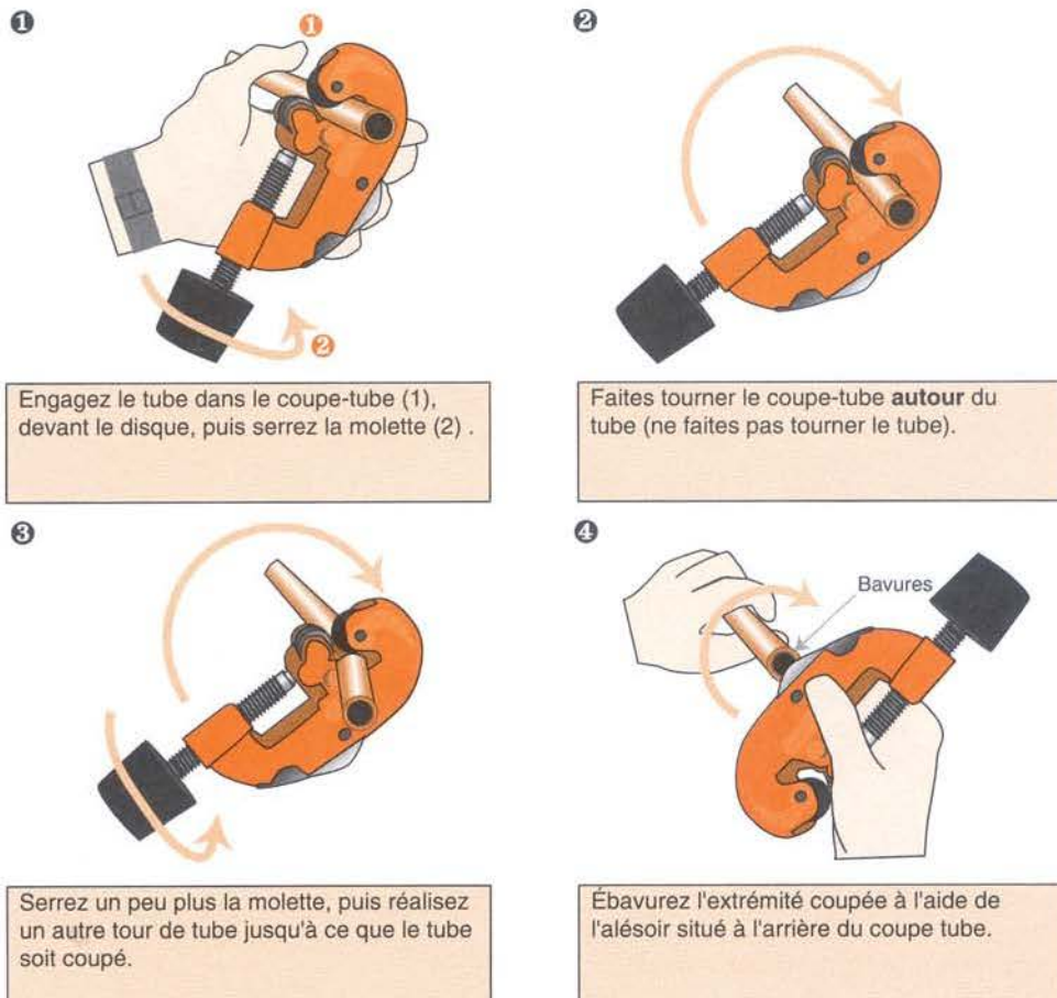
Figure 105 : L'utilisation du coupe-tube
