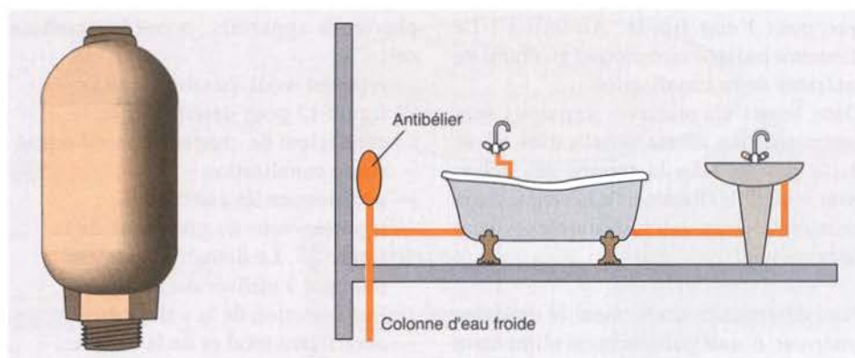
Figure 16 : L'antibélier
