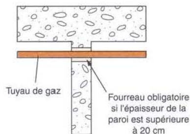
Traversée de murs ou cloisons
