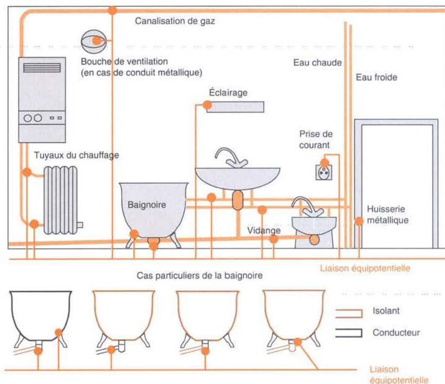
Figure 71 : La liaison équipotentielle
