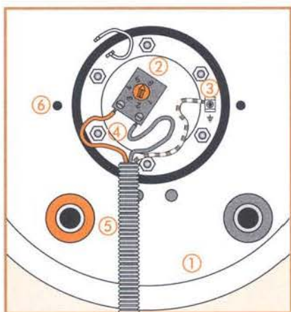
Figure 145 : Le raccordement électrique d'un chauffe-eau
