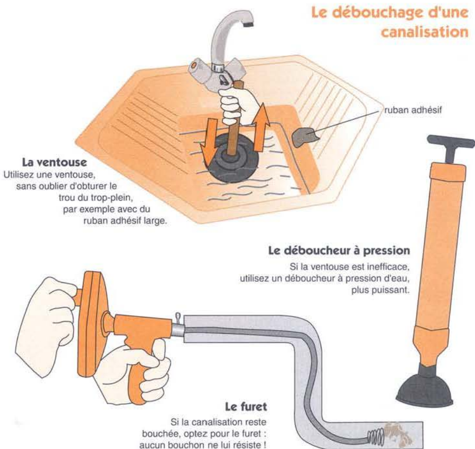
Figure 150 : Le débouchage d'un évier ou d'un lavabo
