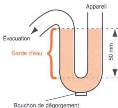
Figure 20 : Le siphon
