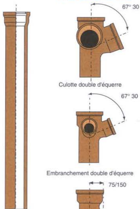
Tuyau fonte SME
