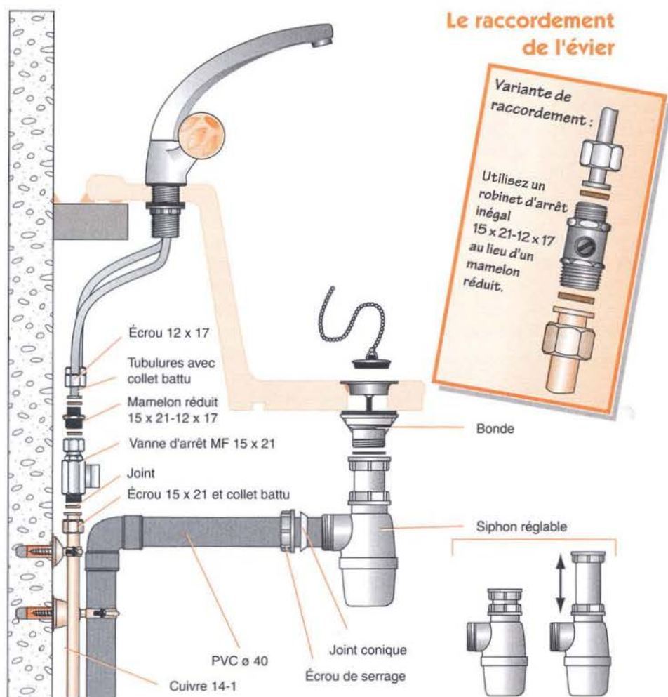
Figure 125 : Le raccordement des évier aux canalisations
