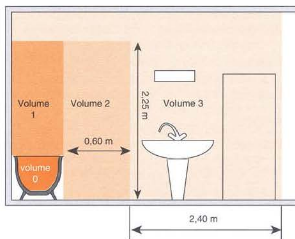
Figure 70 : Les volumes de protection électrique de la salle de bains
