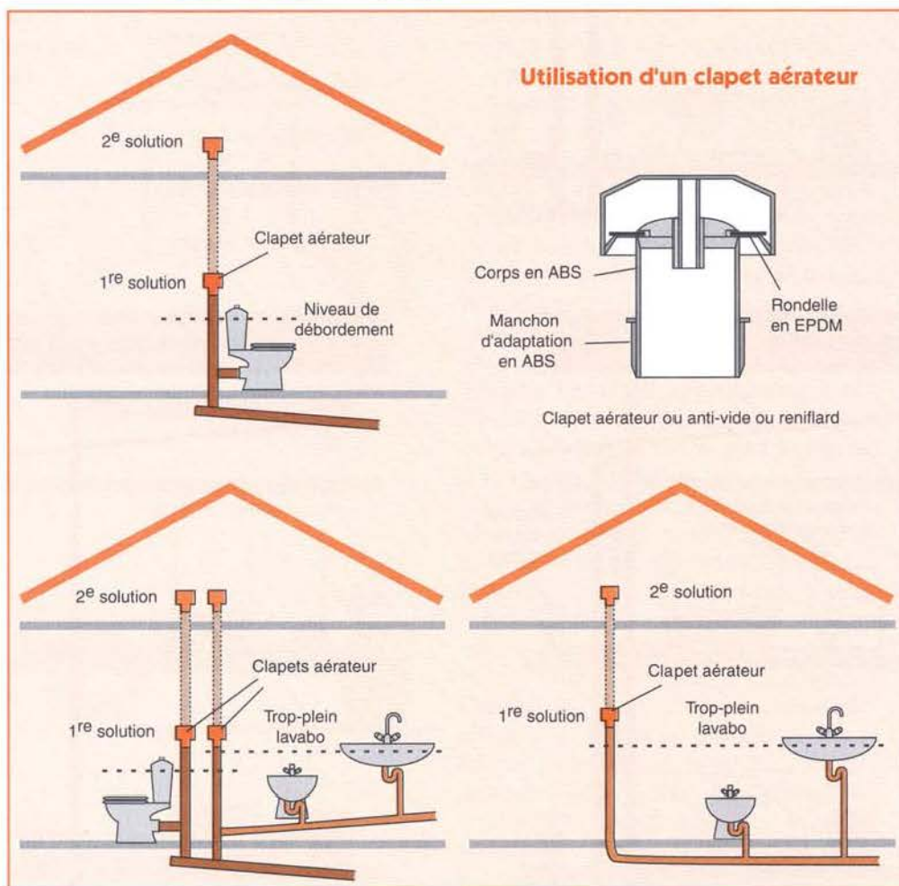
Figure 23 : Le clapet aérateur
