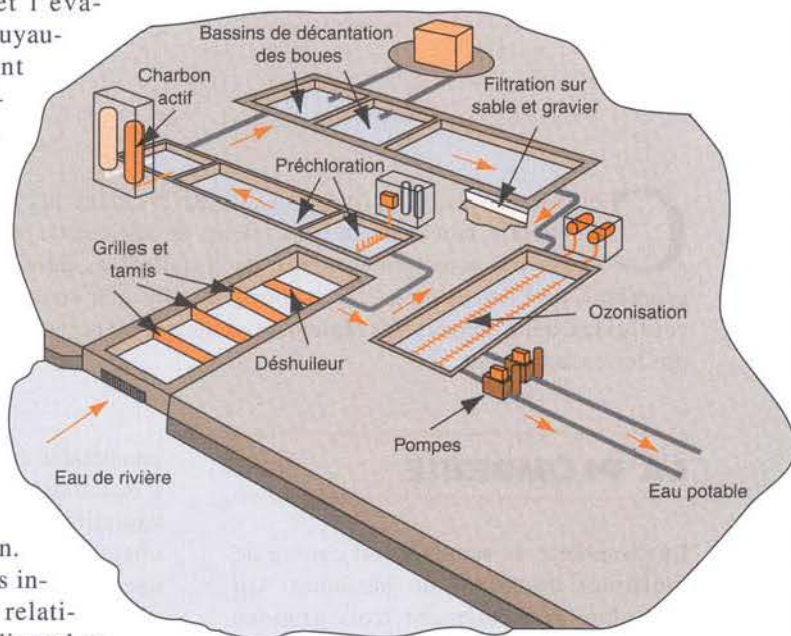
Figure 1 : L'épuration de l'eau
