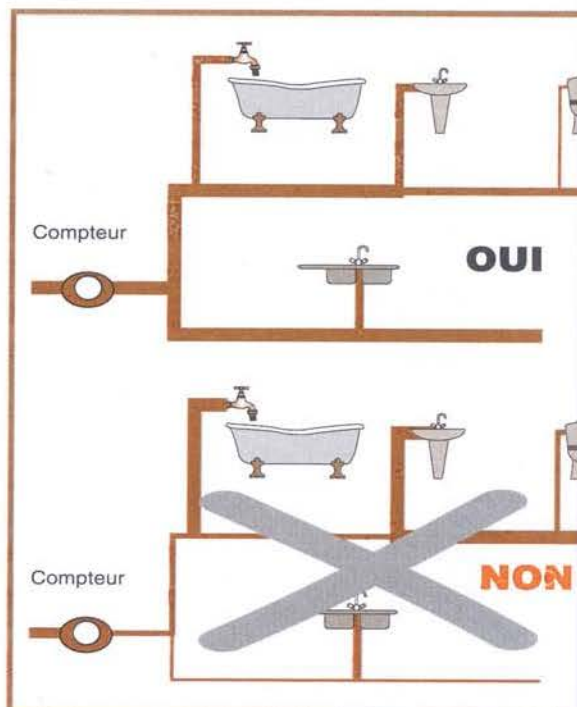
Figure 3 : Le principe de réduction des diamètres
