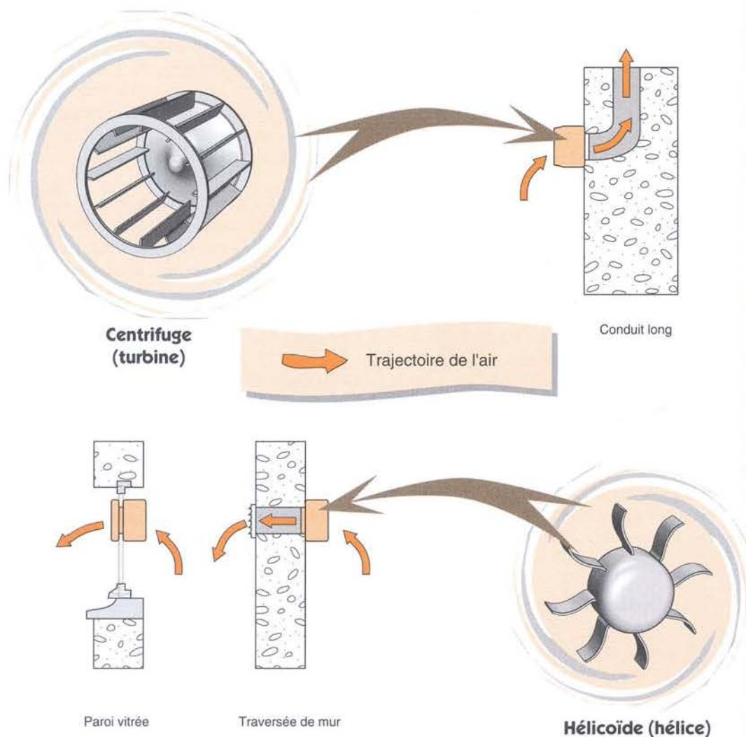
Figure 65 : Les aérateurs
