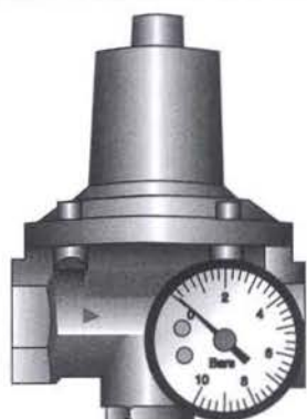
Réducteur de pression réglable avec manomètre de contrôle
