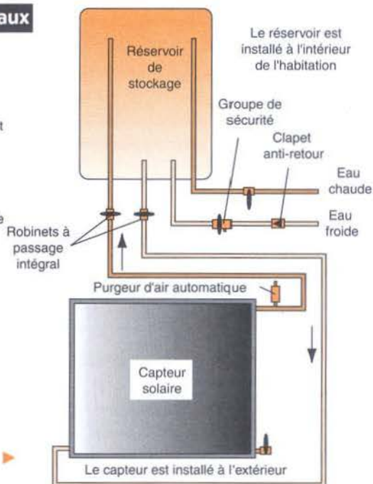
Chauffe-eau thermosiphon à éléments séparés
