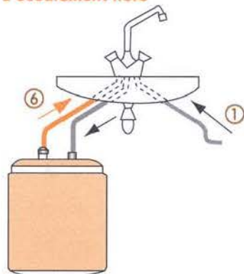
Figure 144 : Les divers raccordements hydrauliques
