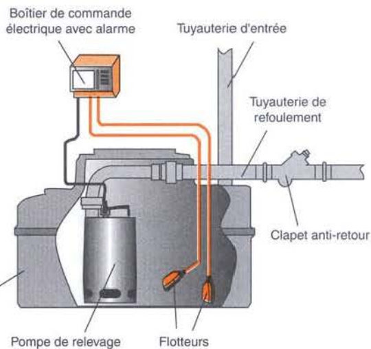
Figure 26 : Le relevage des eaux usées
