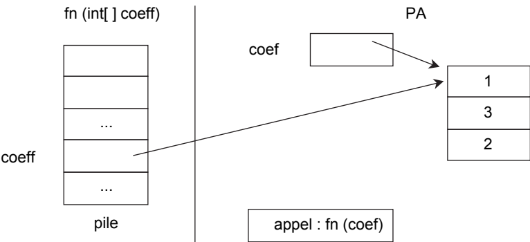
Figure 1.10 — Le passage par adresse du tableau : on recopie dans la pile, l’adresse (la référence) du tableau coef . La modification d’un élément du tableau coeff dans la fonction ( coeff[1]=4 ) se répercute dans le programme appelant. Voir le programme Java ci-dessous.
