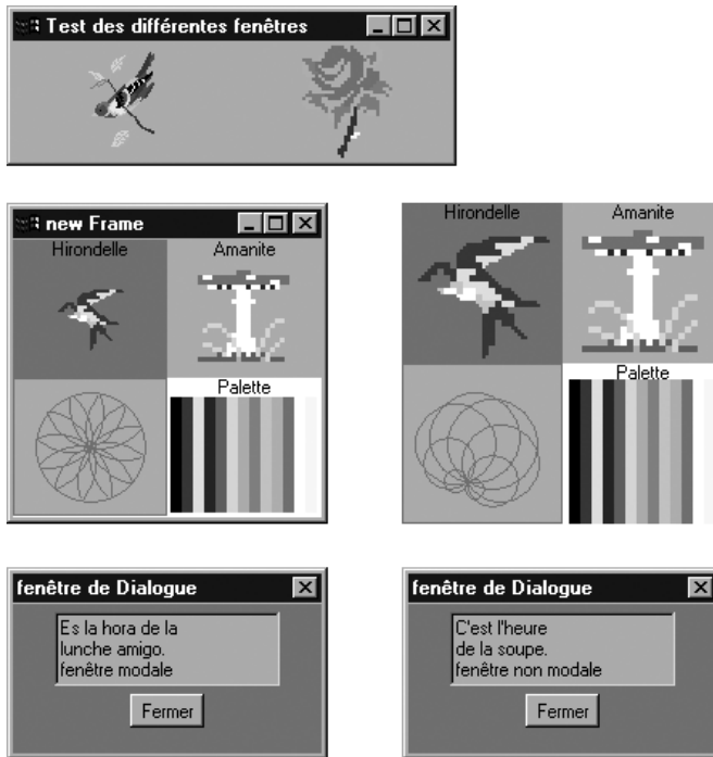
Figure 5.38 — Les différents types de fenêtres : Frame, Window et Dialog.
