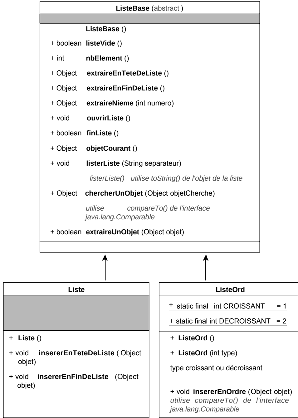
Figure 4.1 — Arbre d'héritage des listes (vue utilisateur).
