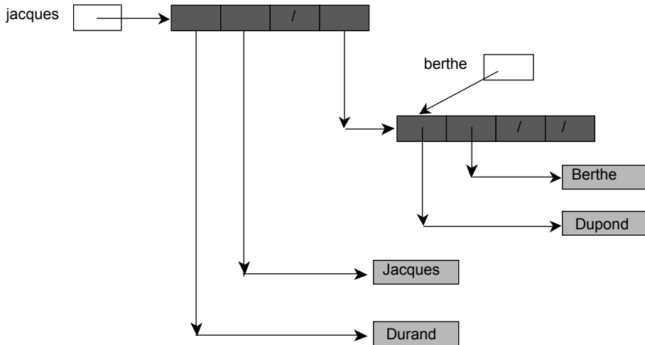
Figure 2.15 — L'implémentation des références en Java (deux objets de type Personne , quatre objets de type String ).
