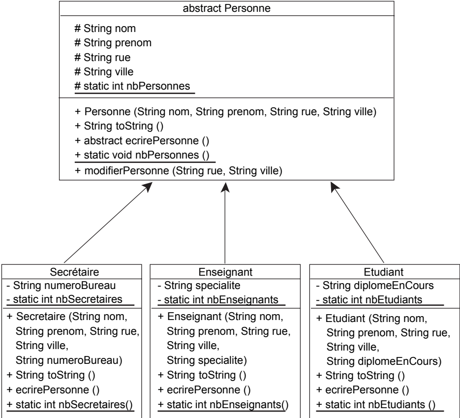
Figure 3.2 — Arbre d’héritage.
