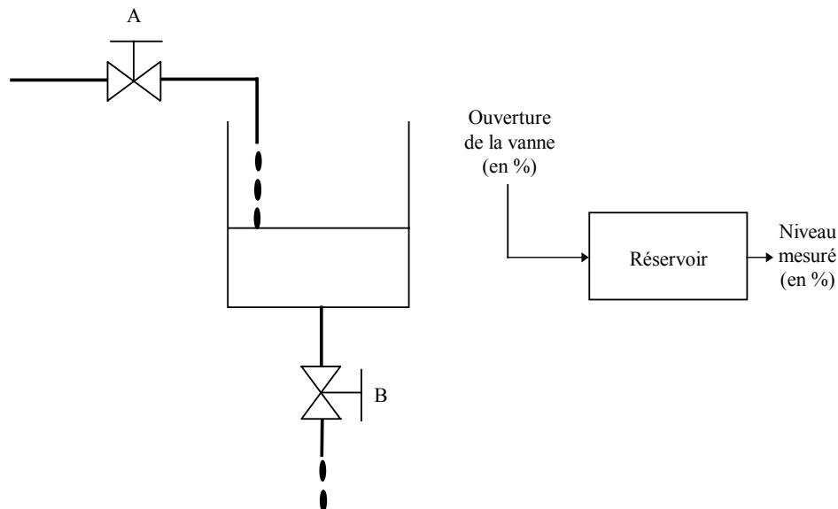
Figure 6-15 Réservoir simple
