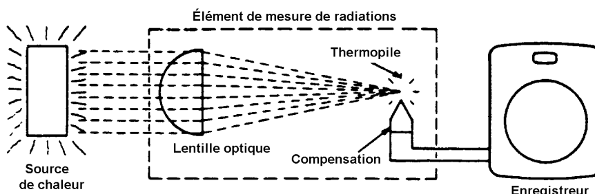
Figure 5-69 : Thermomètre mesurant les radiations
