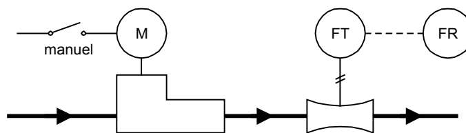
Figure 2-30 Schéma de principe d'un procédé de débit
