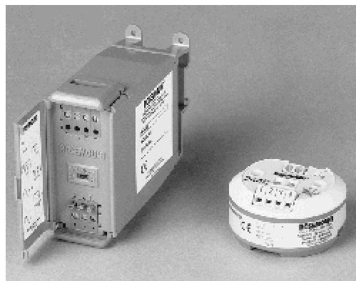
Figure 3-2 Transmetteurs
