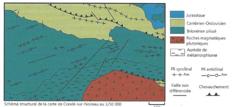
▲ Schéma structural de la carte de Condé-sur-Noireau. D'après BORDI et al. (2018)
