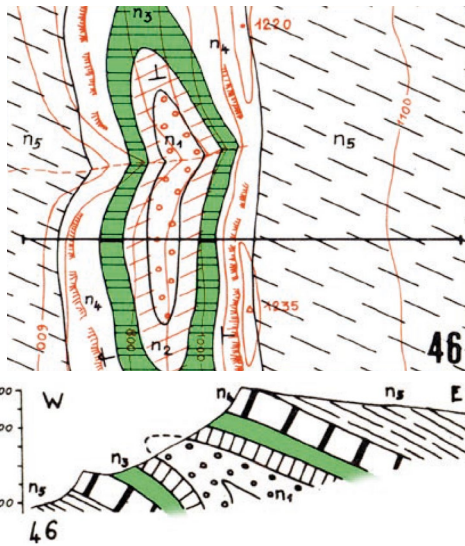
▲ Pli anticlinal. D'après FOUCAULT & RAOULT (1966) modifié par B. ANSELME (BCPST2, Lycée Fénelon, Paris)
