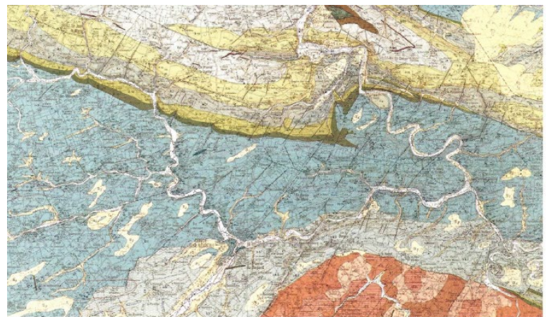
▲ Carte de Condé-sur-Noireau. D'après BORDI et al. (2018)
