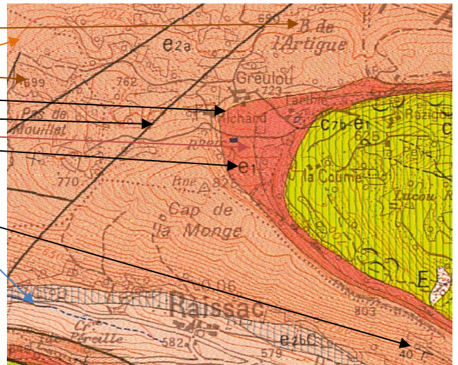
▲ Extrait de la carte au 1/50000 de Lavelanet. © BRGM.
