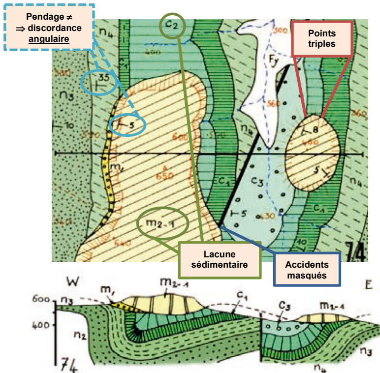
▲ Indices d'une discordance . D'après FOUCAULT & RAOULT (1966) modifié par B. ANSELME (BCPST2, Lycée Fénélon, Paris)
